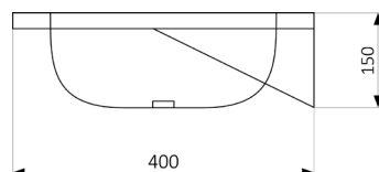
SLM 1AT – widok z boku
