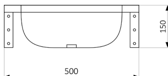
SLM 1AT – widok z przodu
