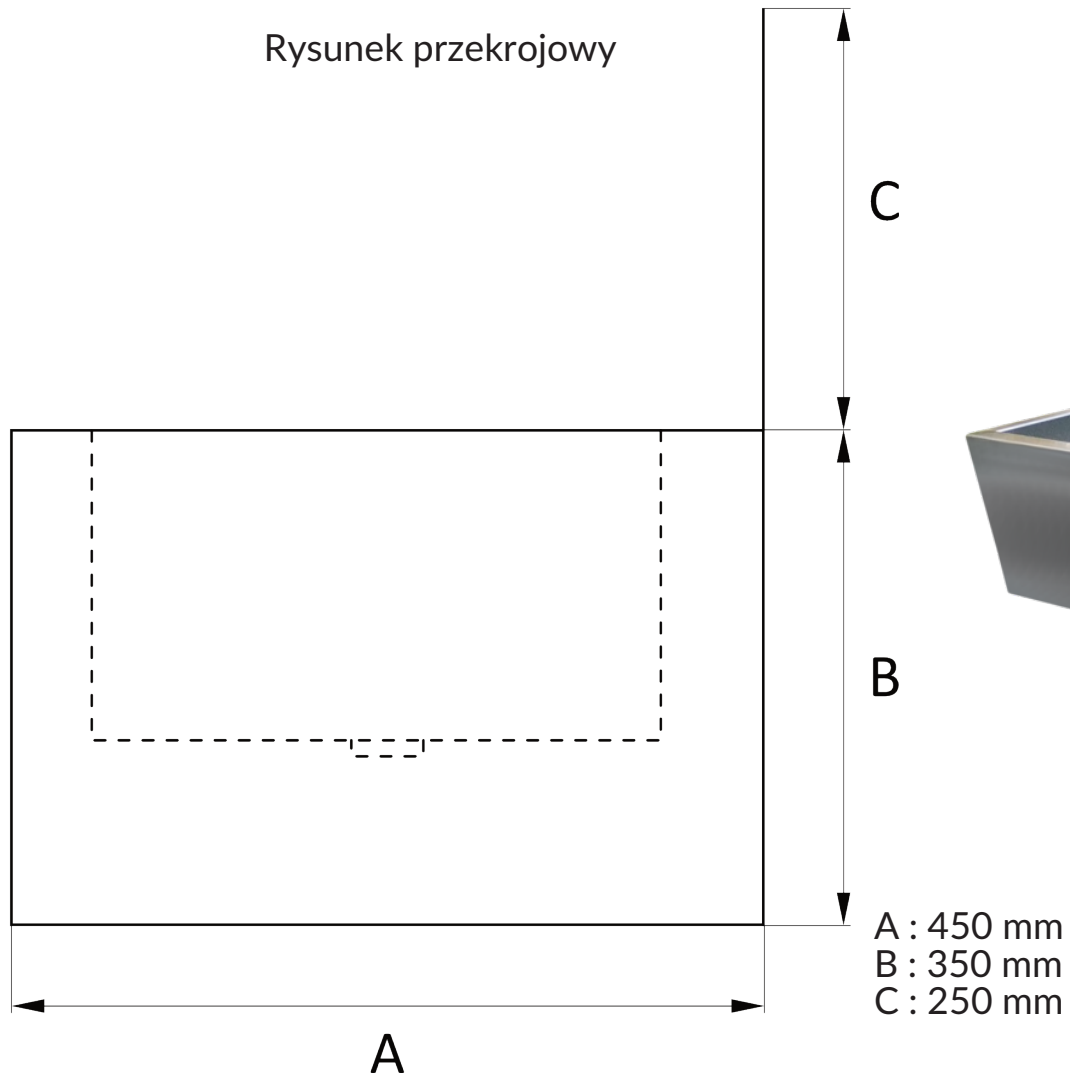
Umywalka rynnowa z osłoną syfonu i ściany
